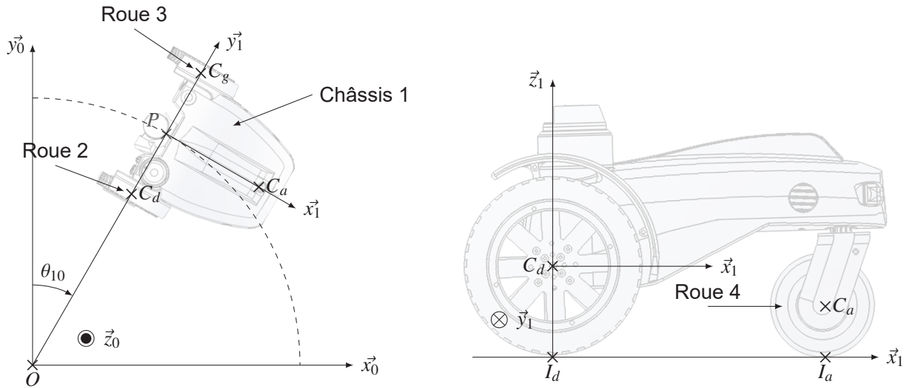
Figure 6 - Paramétrage du Bering avec une roue folle
