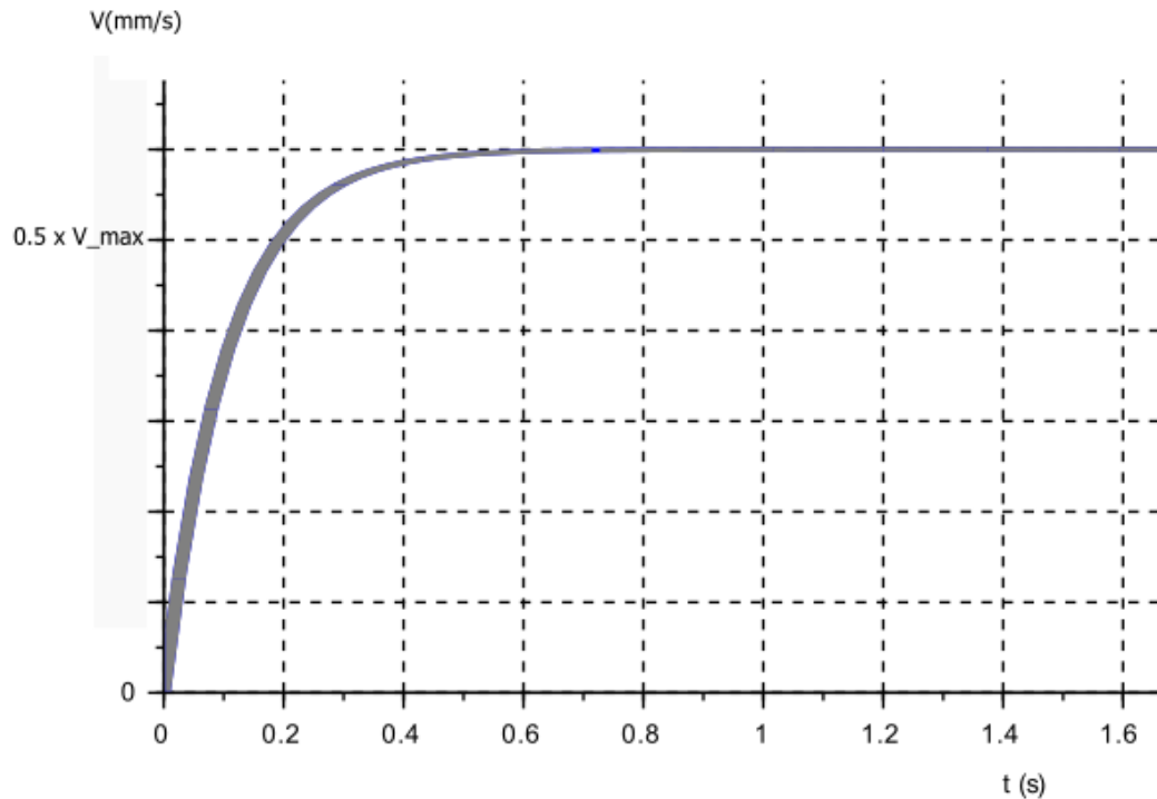
Figure 17 - Simulation de la boucle de vitesse
