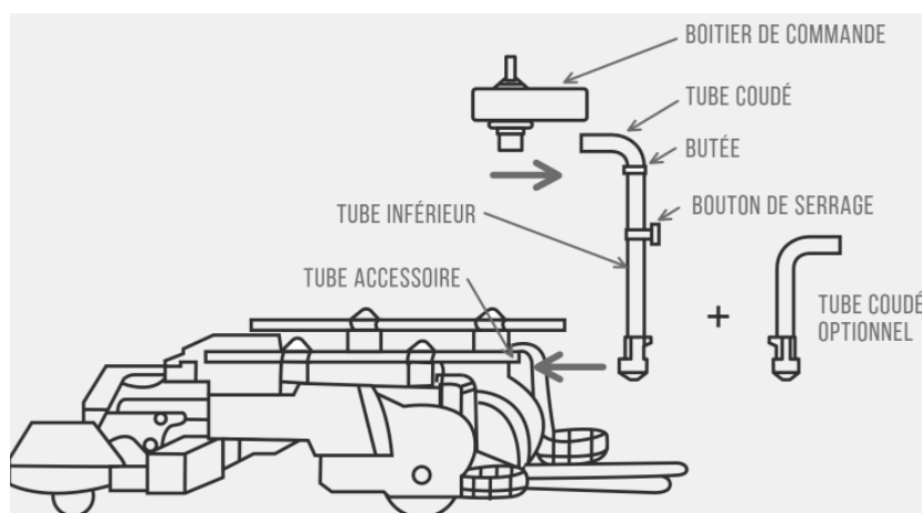
Figure 2 - Représentation schématique du Mobilikit
