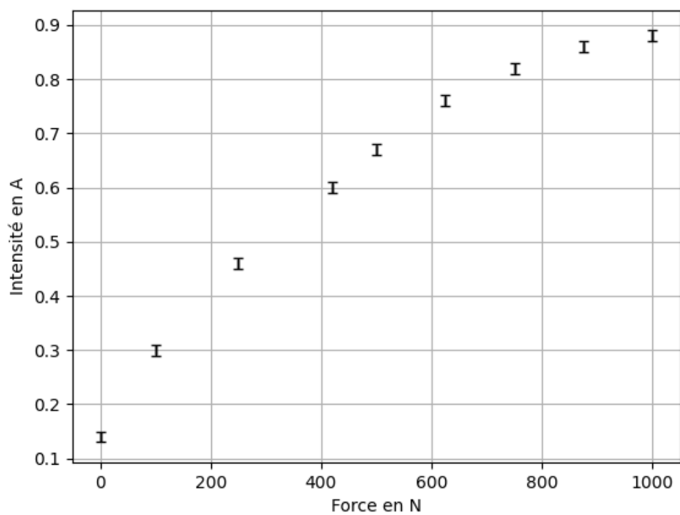
Figure 6 - Courbes d'évolution de la vitesse de translation de la tige du vérin v et du courant absorbé I en fonction de la force F_{\text{vérin}}
