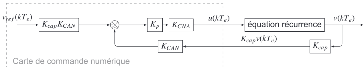
Figure 16 - Schéma-bloc de la boucle de vitesse avec commande numérique
