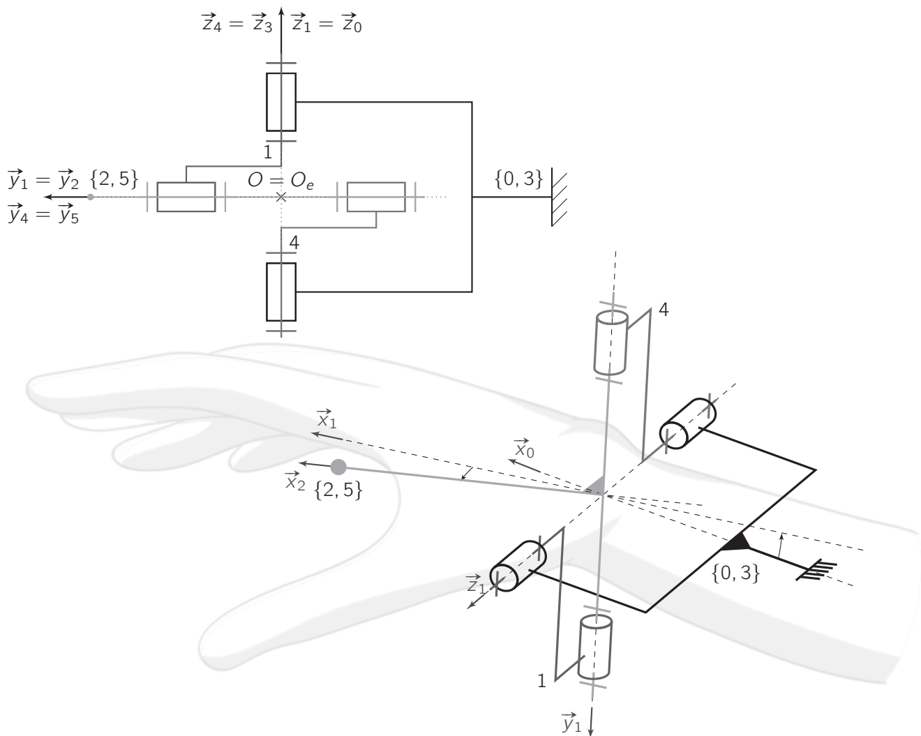
Figure 7 – Schémas cinématiques du bras et de l'exosquelette dans le cas où \mathcal{R}_4 = \mathcal{R}_1
