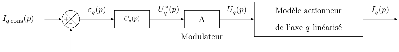
Figure 13 Modèle linéarisé de la boucle d'asservissement du courant i_q
