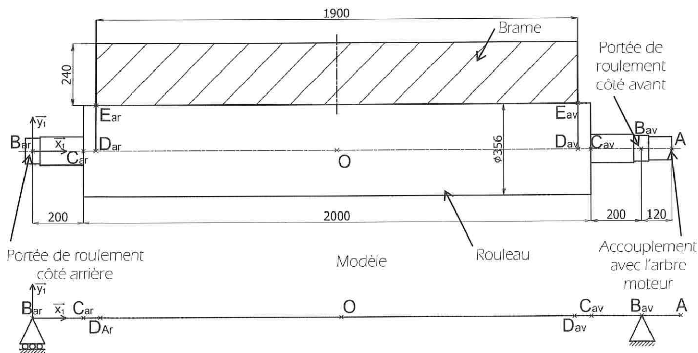
Figure 10 - Dessin d'un rouleau et modèle associé
