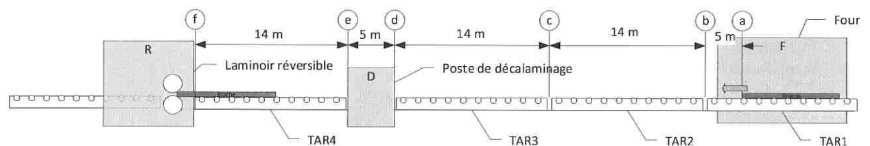
Figure 17 - Implantation actuelle de la ligne
