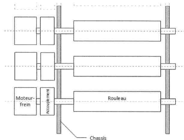
Figure 7 - Motorisation modulaire des rouleaux
