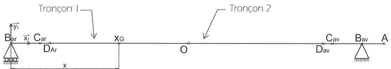
Figure 12 - Paramétrage de la poutre
