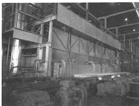
Figure 5 - Brame chaude à la sortie du four à brame
