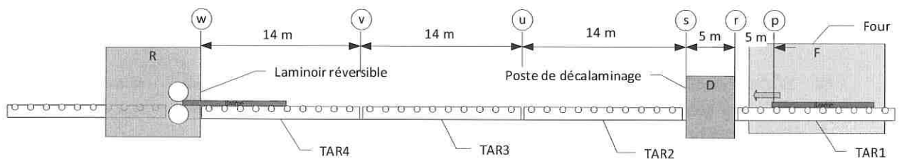
Figure 18 - Implantation envisagée de la ligne
