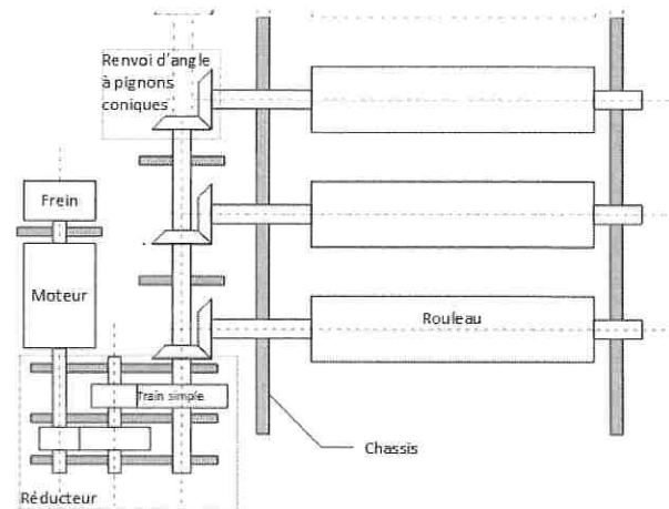
Figure 6 - Motorisation actuelle des rouleaux
