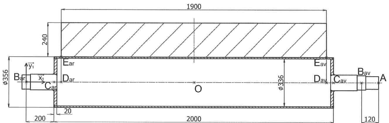
Figure 14 - Dessin du rouleau creux envisagé
