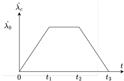
Figure 27 - Consigne de vitesse en trapèze
