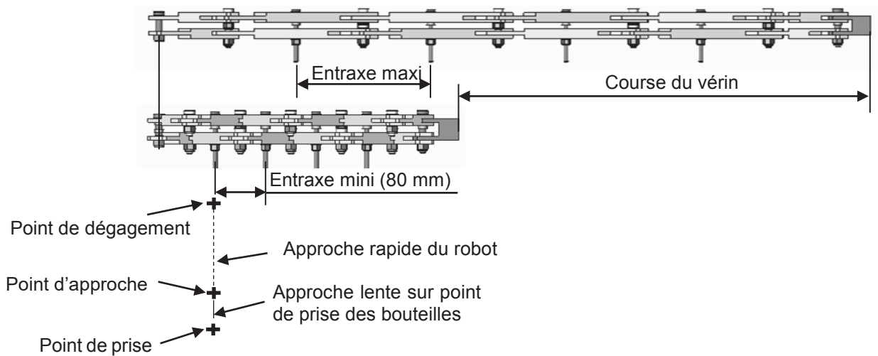
Figure 12 - Positions minimum et maximum du pantographe
