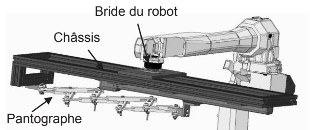
Figure 9 - Châssis support du pantographe
