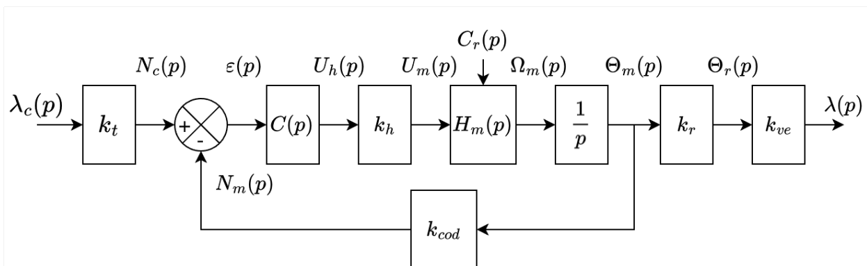
Figure 24 - Schéma-bloc de l'asservissement en position
