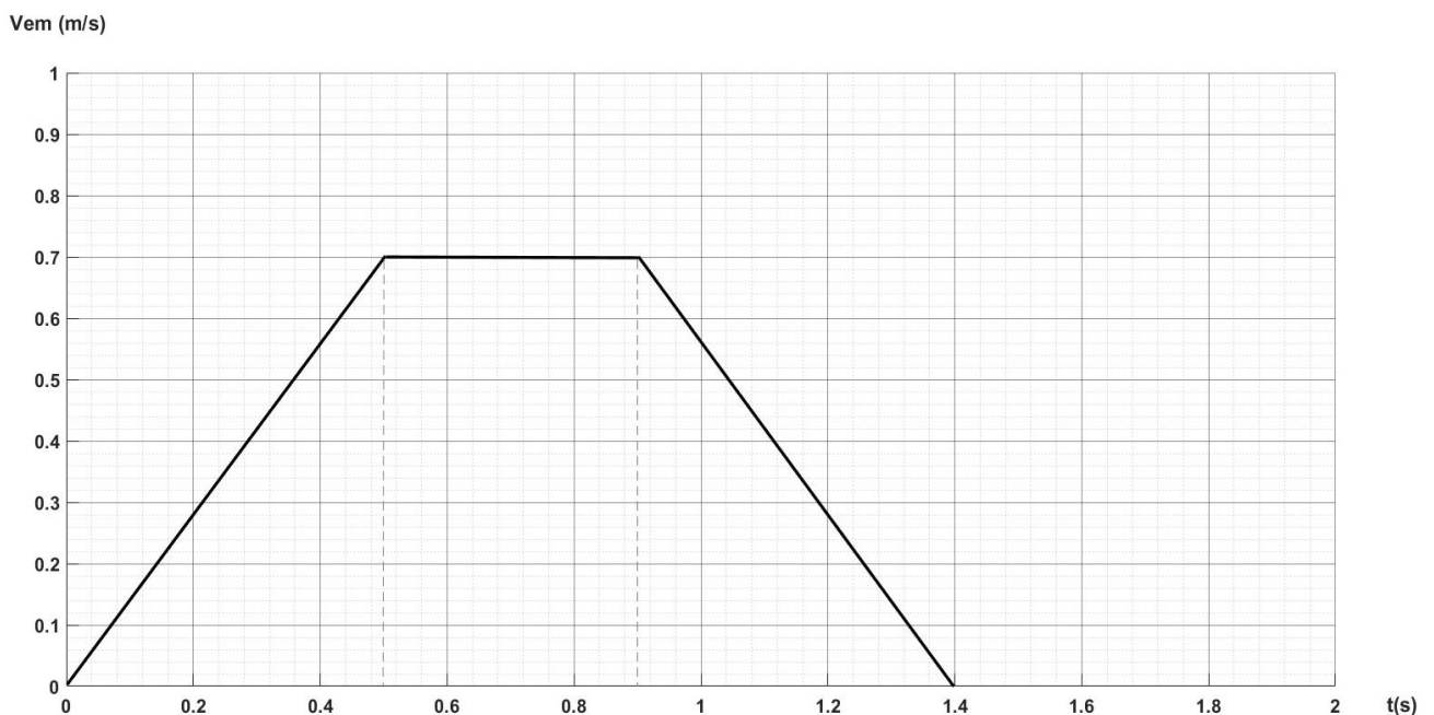
Figure 31 - Vitesse de déplacement du vérin
